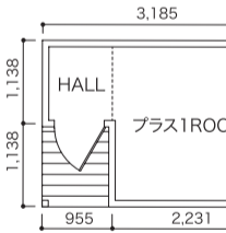
■1R(基本サイズにルームを1延長)
