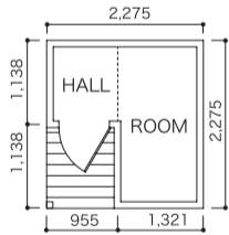
■1H(基本サイズにホールを1延長)
