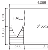
■2R(基本サイズにルームを2延長)
