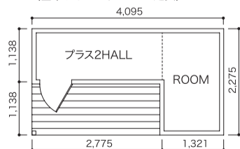
■2H(基本サイズにホールを2延長)
